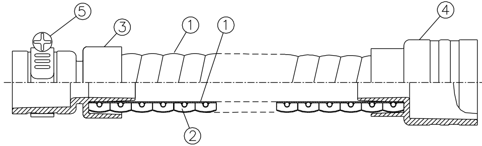
継手付き断熱ドレンホース DSH-FC20S30S
