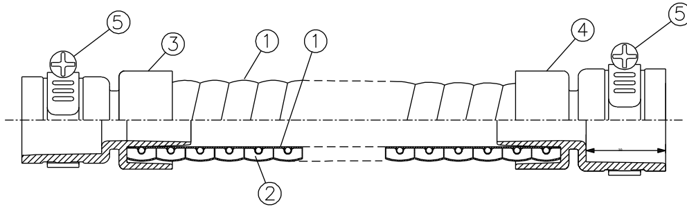
継手付き断熱ドレンホース DSH-FC20S20S/DSH-FC20S25S
