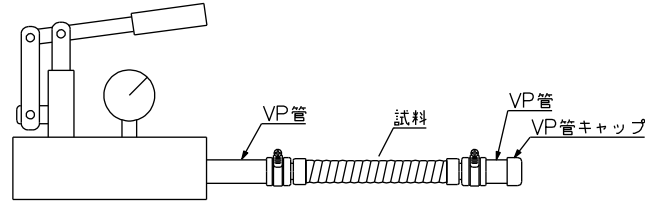
図-1 耐圧試験
