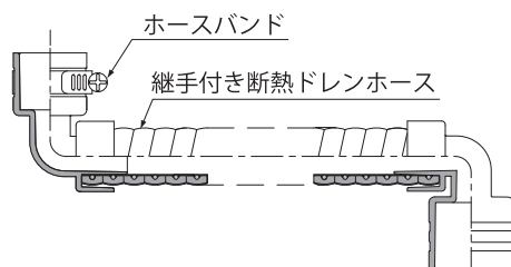
継手付き断熱ドレンホース・・・1 本 (ホースバンド・・・1 個付き)
