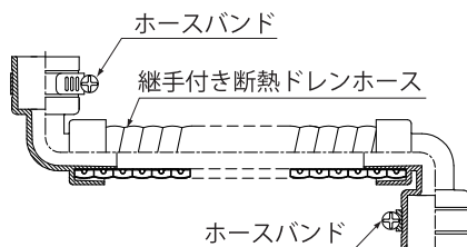
継手付き断熱ドレンホース…1 本 (ホースバンド…2 個付き)
