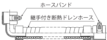
継手付き断熱ドレンホース…1 本 (ホースバンド…2 個付き)
