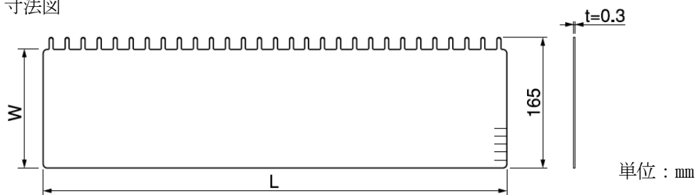
寸法図
