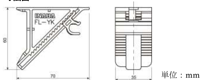
寸法図
