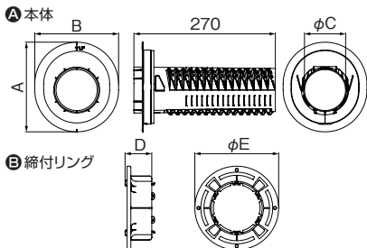
寸法図
