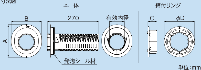
寸法図
