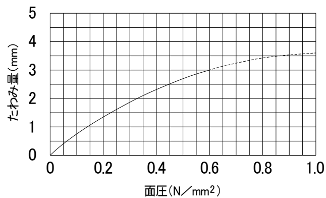
グラフ-2 防振パット GP の面圧-たわみ特性
