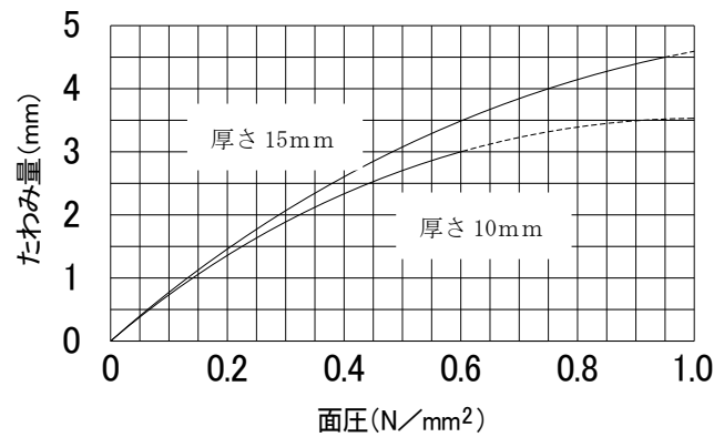
グラフ-1 防振パット GPC の面圧-たわみ特性
