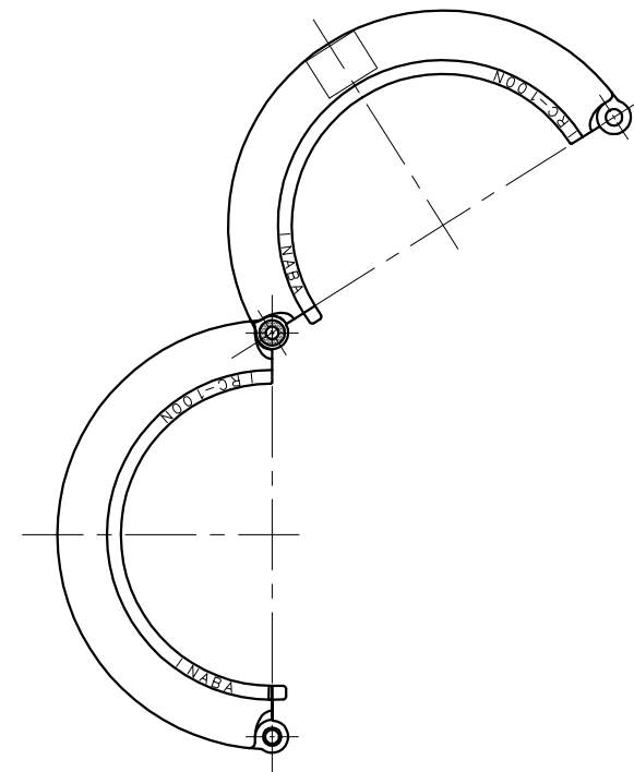
耐火キャップN（乾式壁用）金具可動参考図
