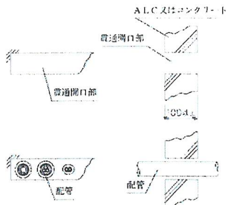
<正面図>
