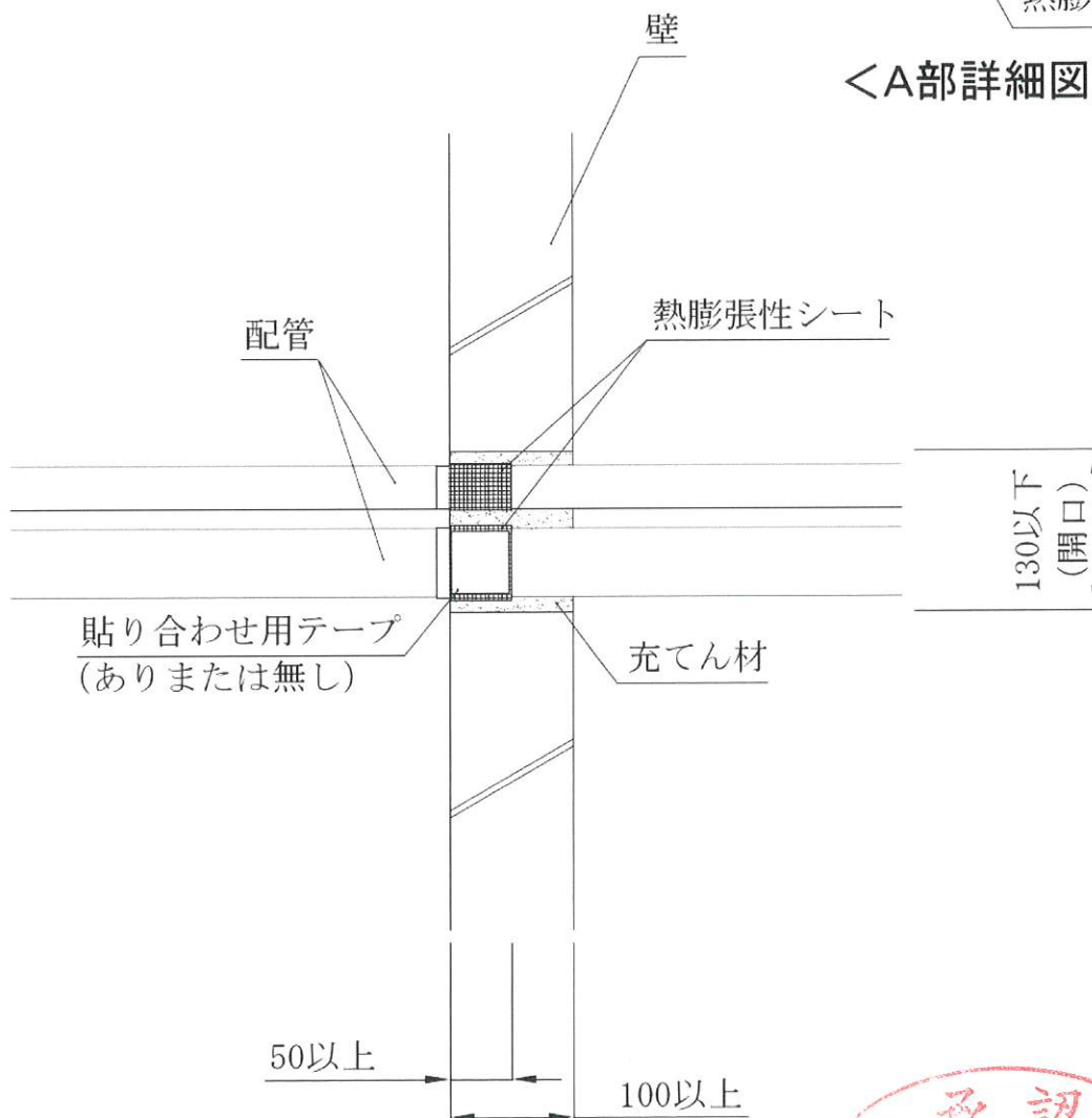
<断面図>
