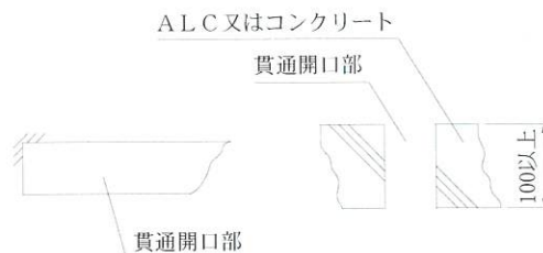
＜正面図＞
