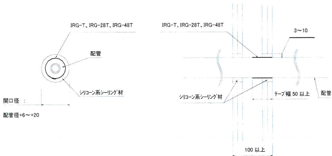
施工断面図
