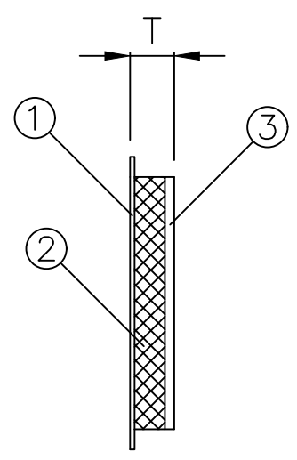
テープ断面
