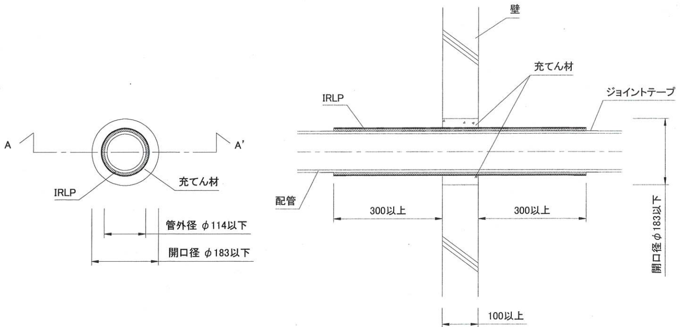
正面図
