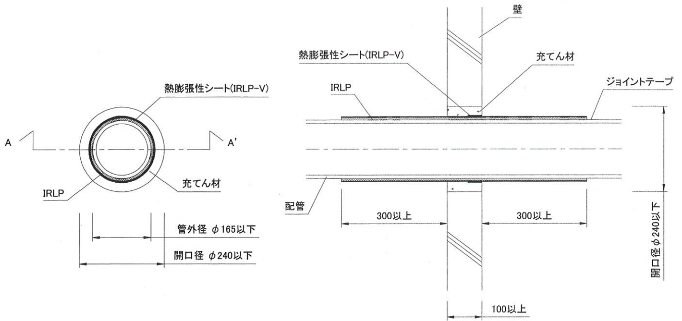
正面図
