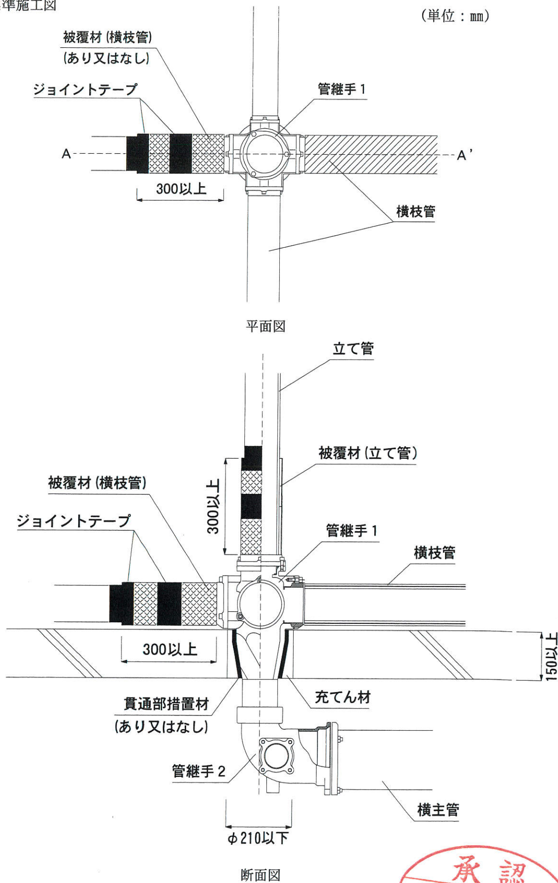
図4 標準施工図
