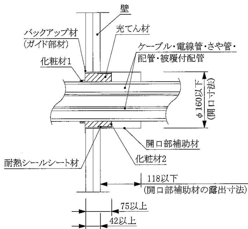
断面図 (高占積率の場合)
