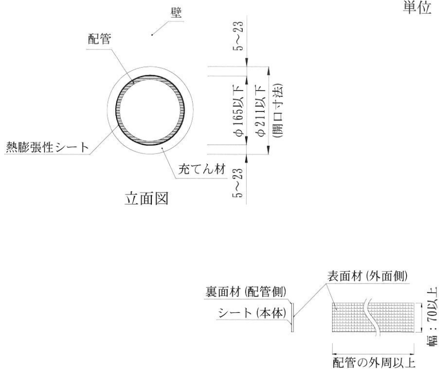
熱膨張性シートの詳細図
