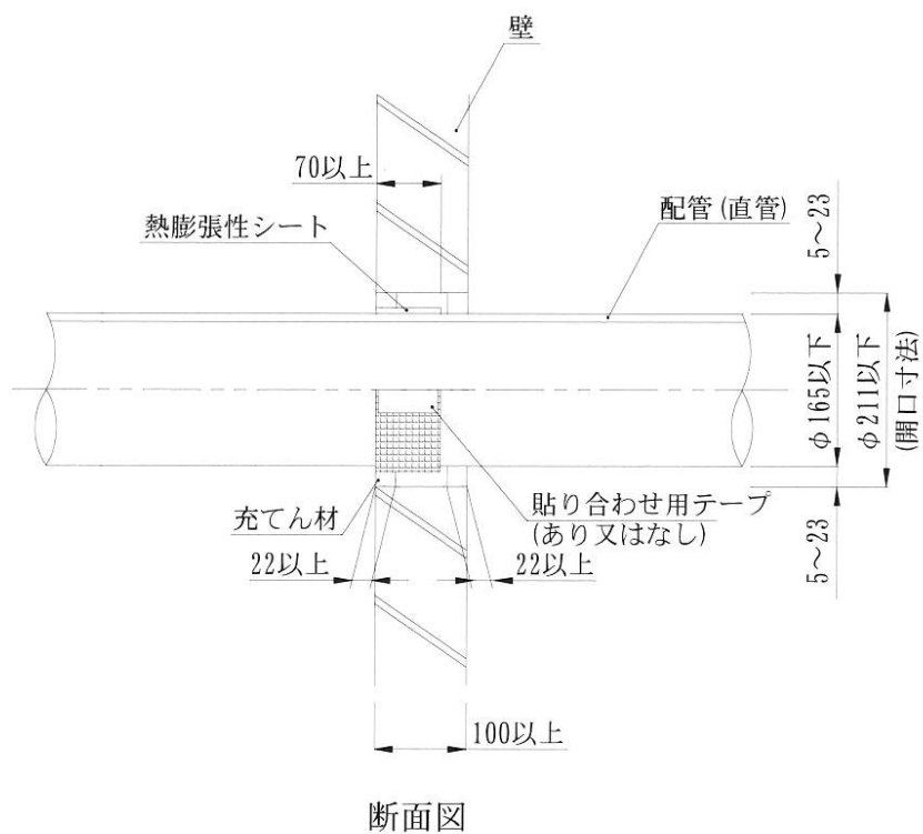
熱膨張性シートの詳細図
