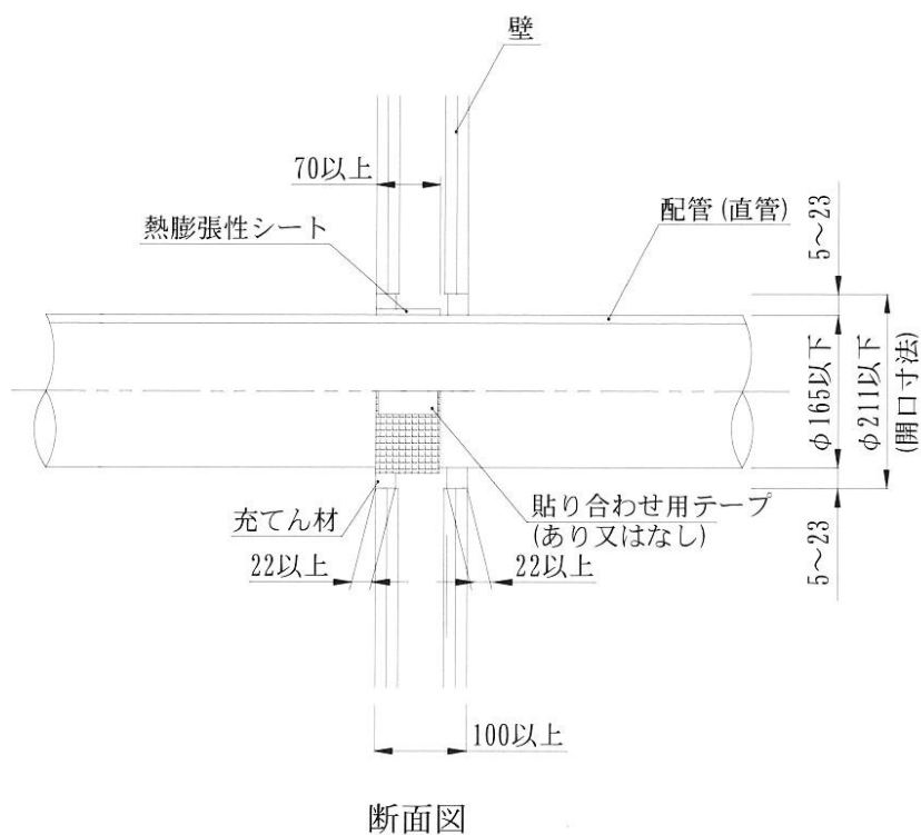
熱膨張性シートの詳細図
