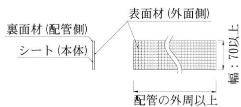
熱膨張性シートの詳細図
