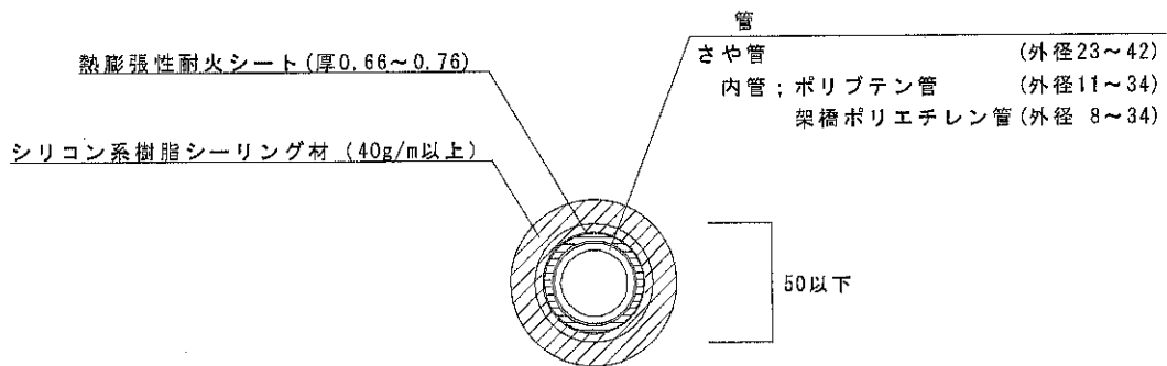
<正面図>
