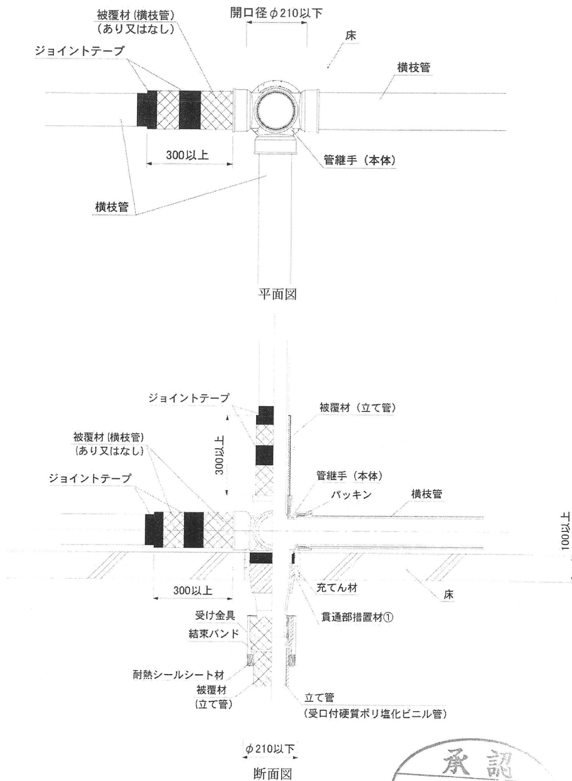
図 6 標準施工図
