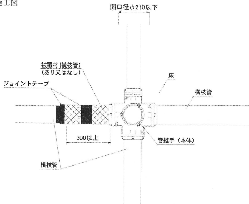
平面図
