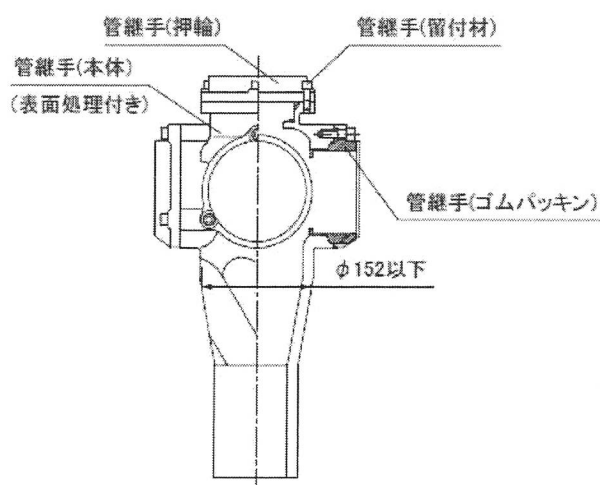
図5 管継手詳細図（代表例）
