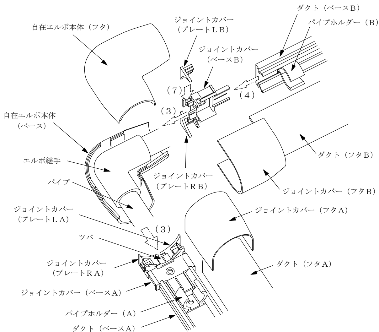
自在エルボ施工図
