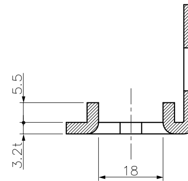
X-X' 断面図
