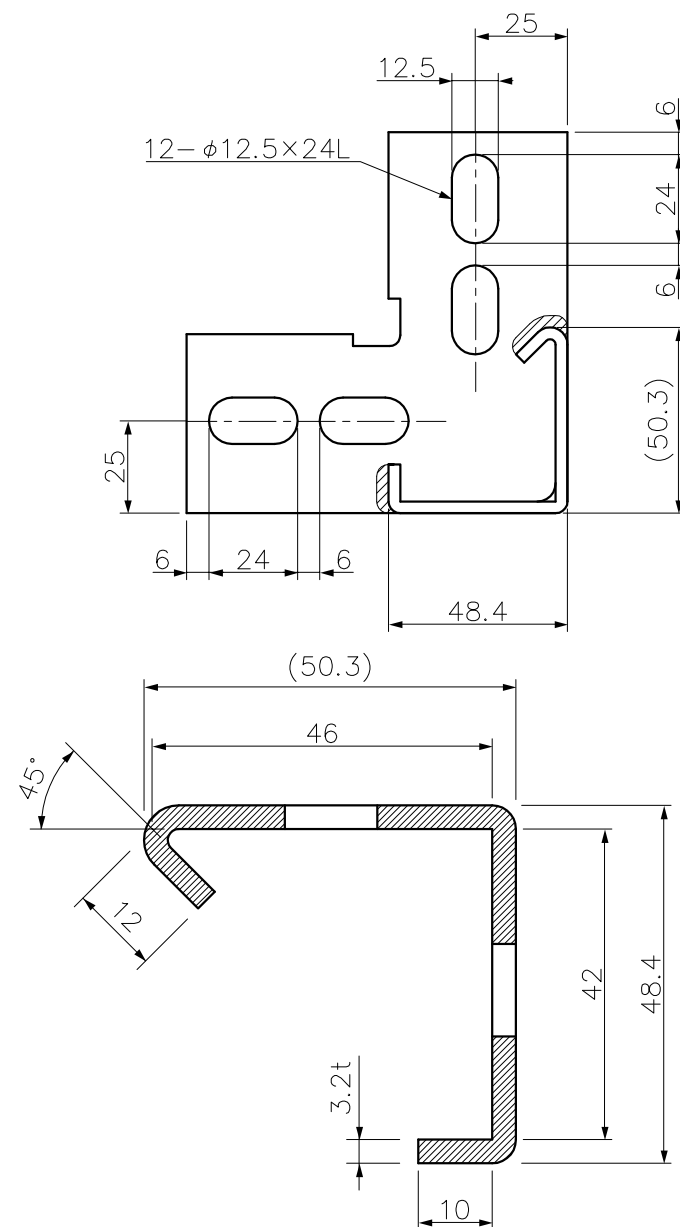
A・B・C・D断面 (S=1/1)
