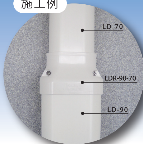
施工例
