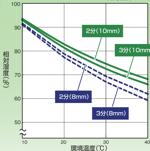
防露性能比較グラフ
