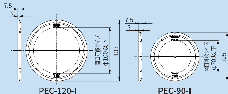
寸法図
