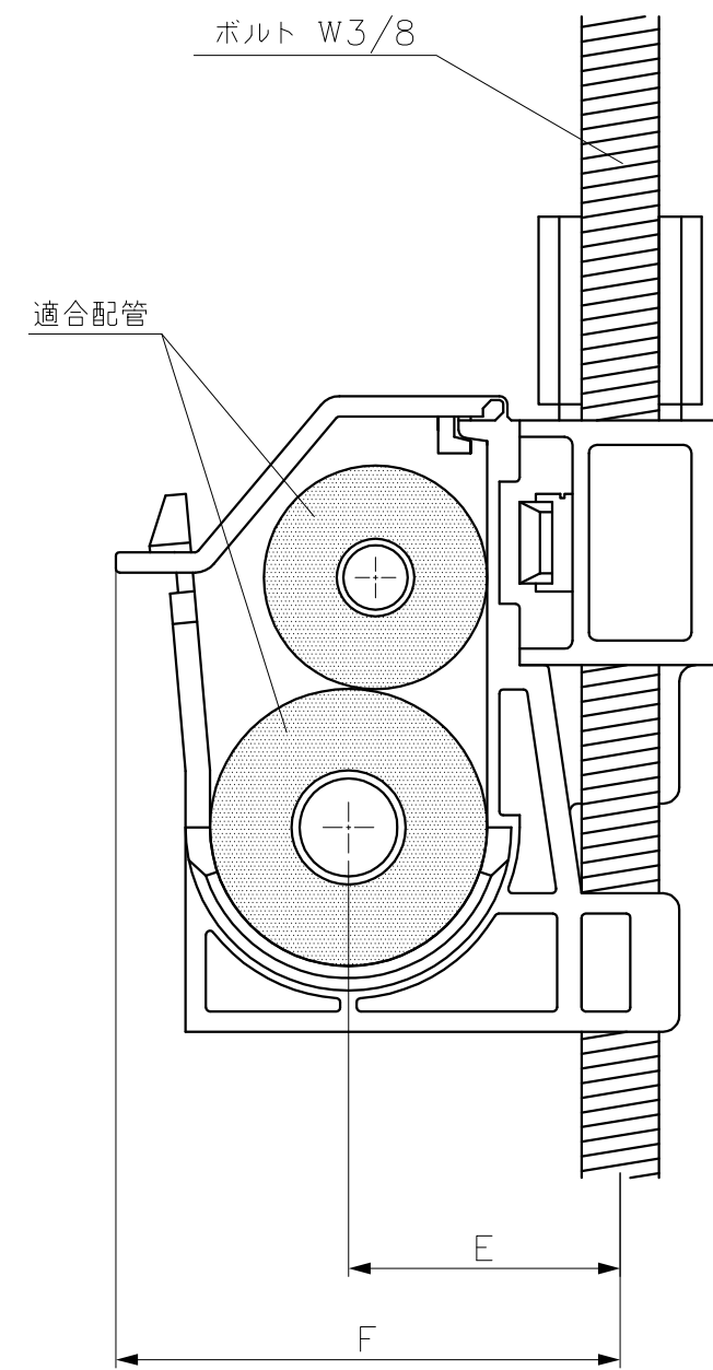
施工図
