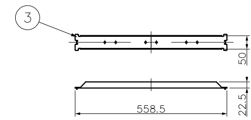
フタ補強板取付位置
