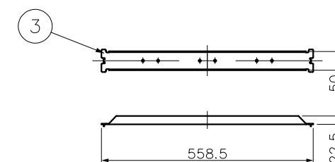
フタ補強板取付位置
