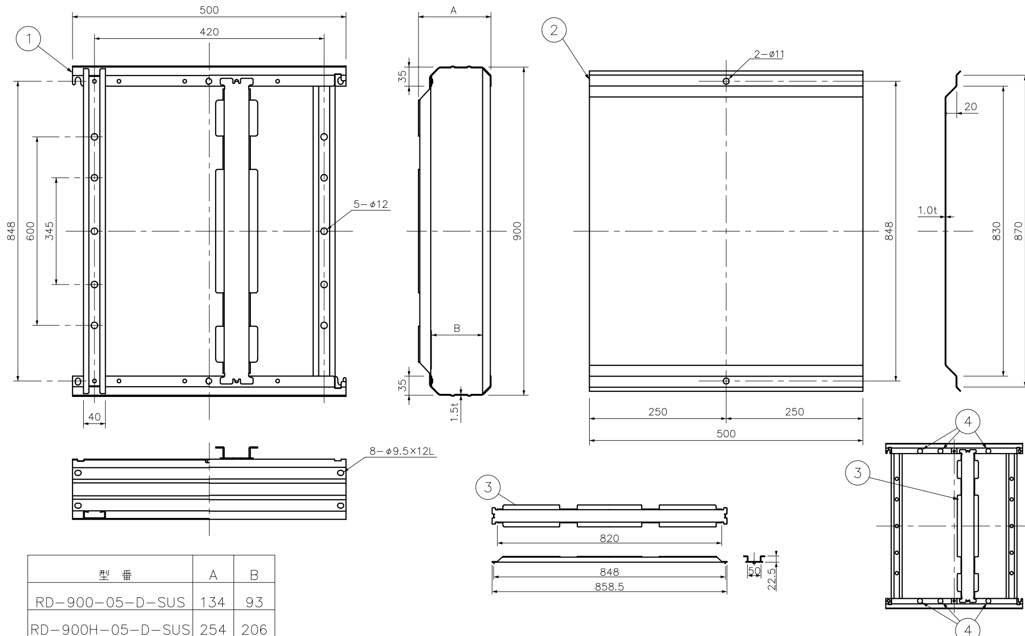
フタ補強板取付位置
