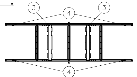
フタ補強板取付位置
