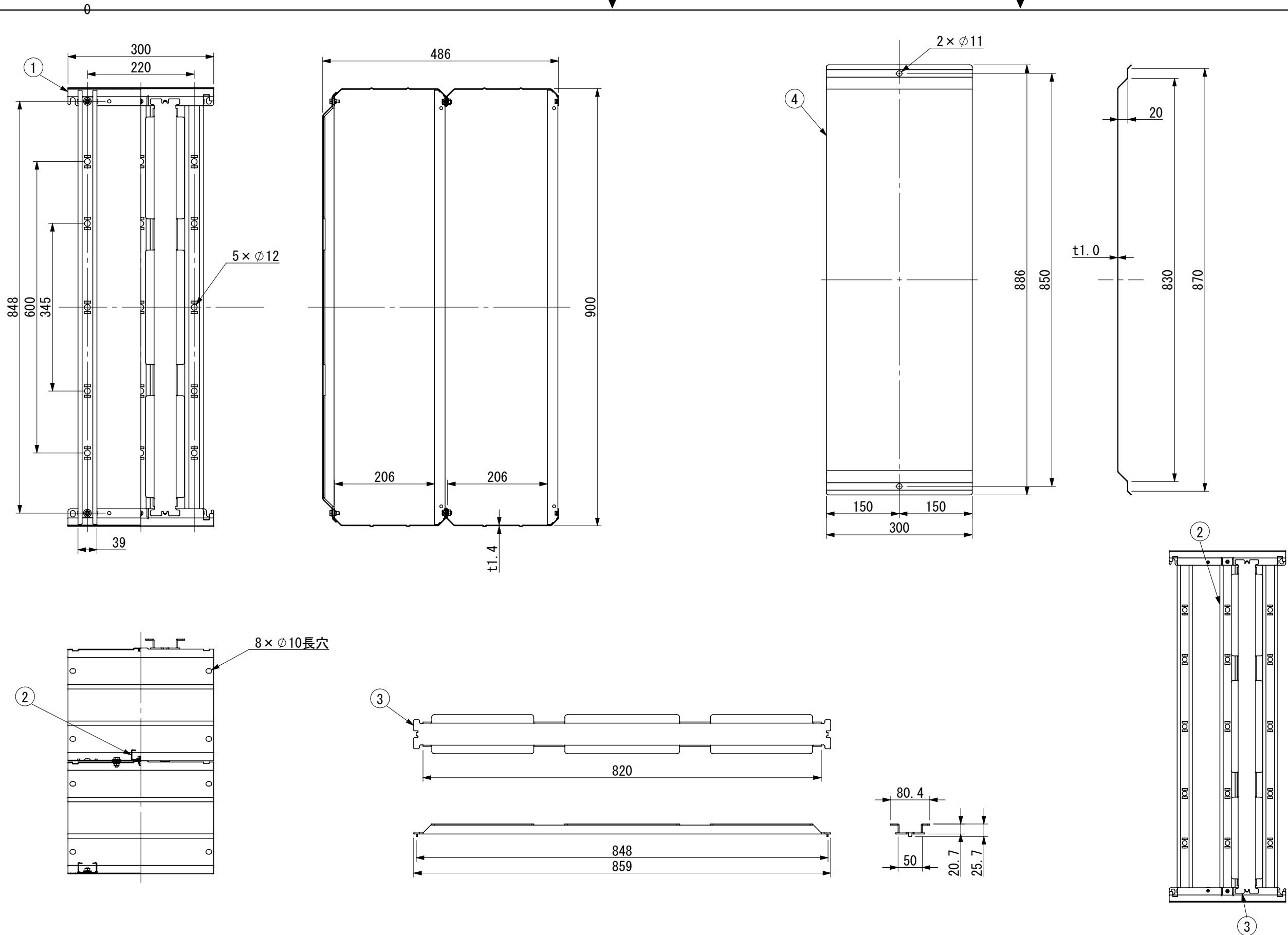
フタ補強板、仕切金具取付位置
