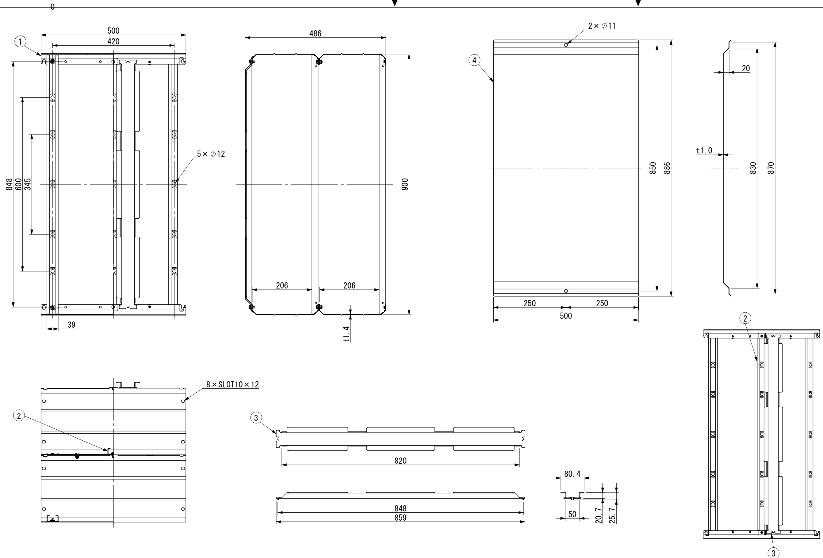
フタ補強板、仕切金具取付位置
