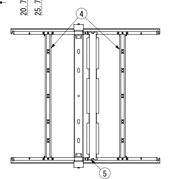
フタ補強板、仕切金具取付位置
