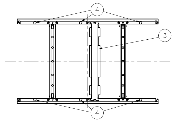
フタ補強板取付位置
