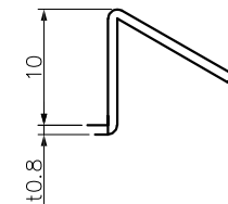
X部詳細 S=2/1
