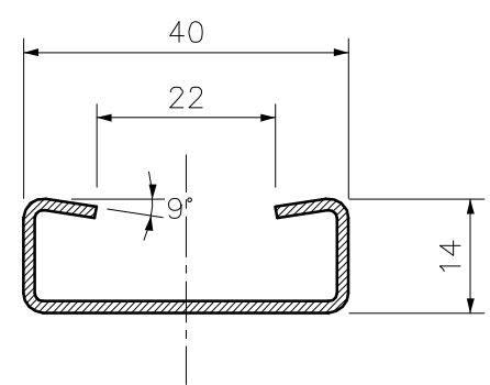
X-X' 断面図 S=1/1
