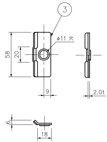
架台固定板
