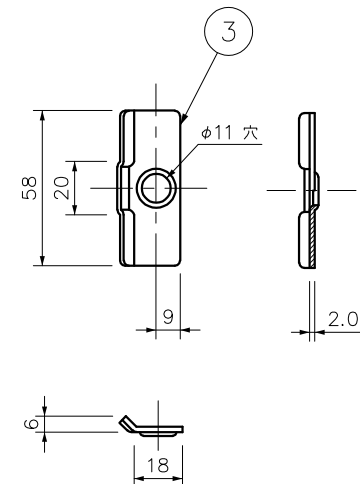
架台固定板
