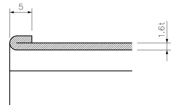
Y部 詳細図 S=2/1
