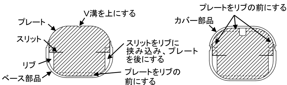
【図1: 取り付け方法】
