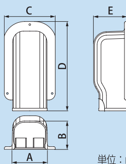
寸法図
