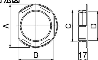
寸法図
