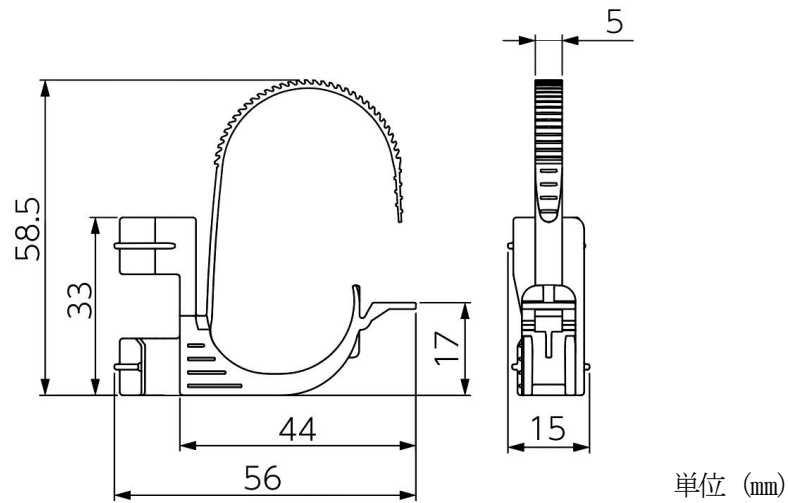
【寸法図】
